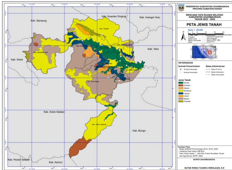
Gambar 2-5 Peta Jenis Tanah Kabupaten Dharmasraya
