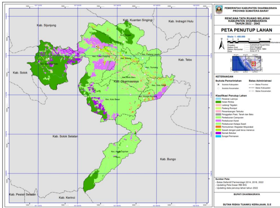
Gambar 2-8 Peta Tutupan Lahan Kabupaten Dharmasraya
