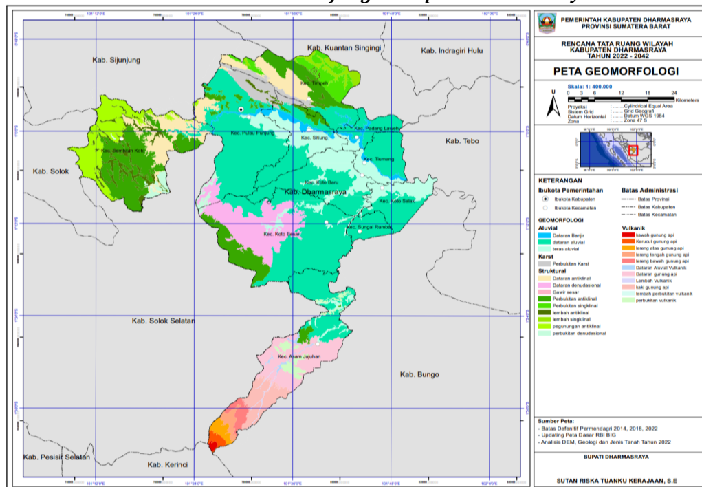
Gambar 2-4 Peta Geomorfologi Kabupaten Dharmasraya
