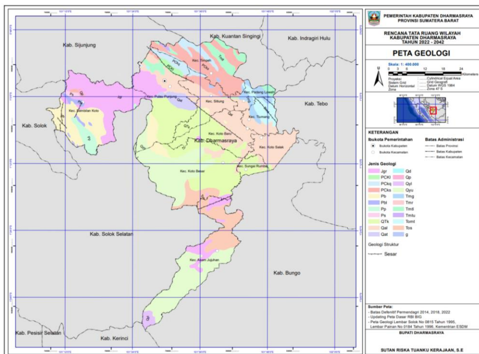
Gambar 2-6 Peta Geologi Kabupaten Dharmasraya
