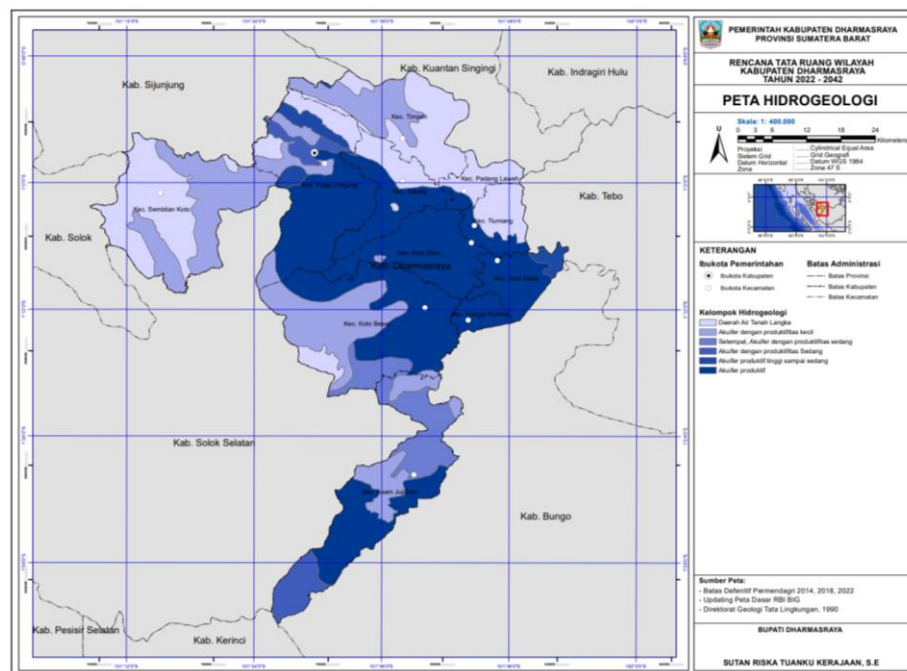
Gambar 2-7 Peta Hidrogeologi Kabupaten Dharmasraya
