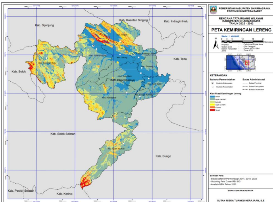
Gambar 2-3 Peta Kelerengan Kabupaten Dharmasraya
