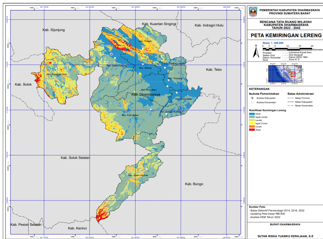
Gambar 2-3 Peta Kelerengn Kabupaten Dharmasraya
