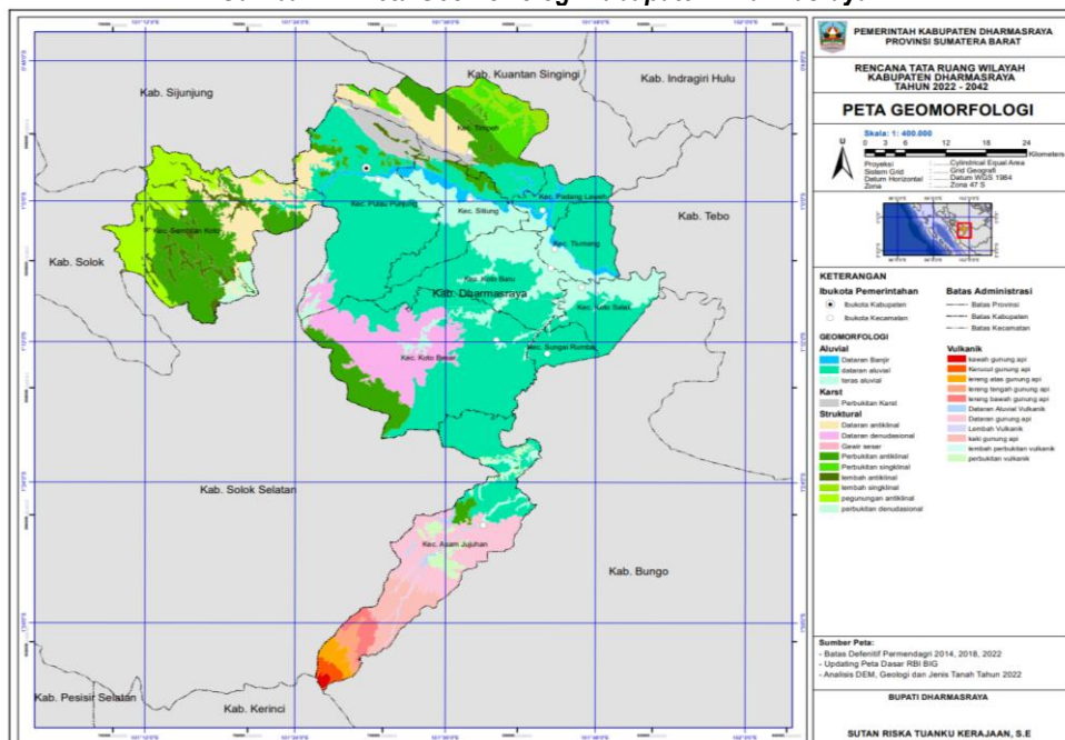
Gambar 2-4 Peta Geomorfologi Kabupaten Dharmasraya
