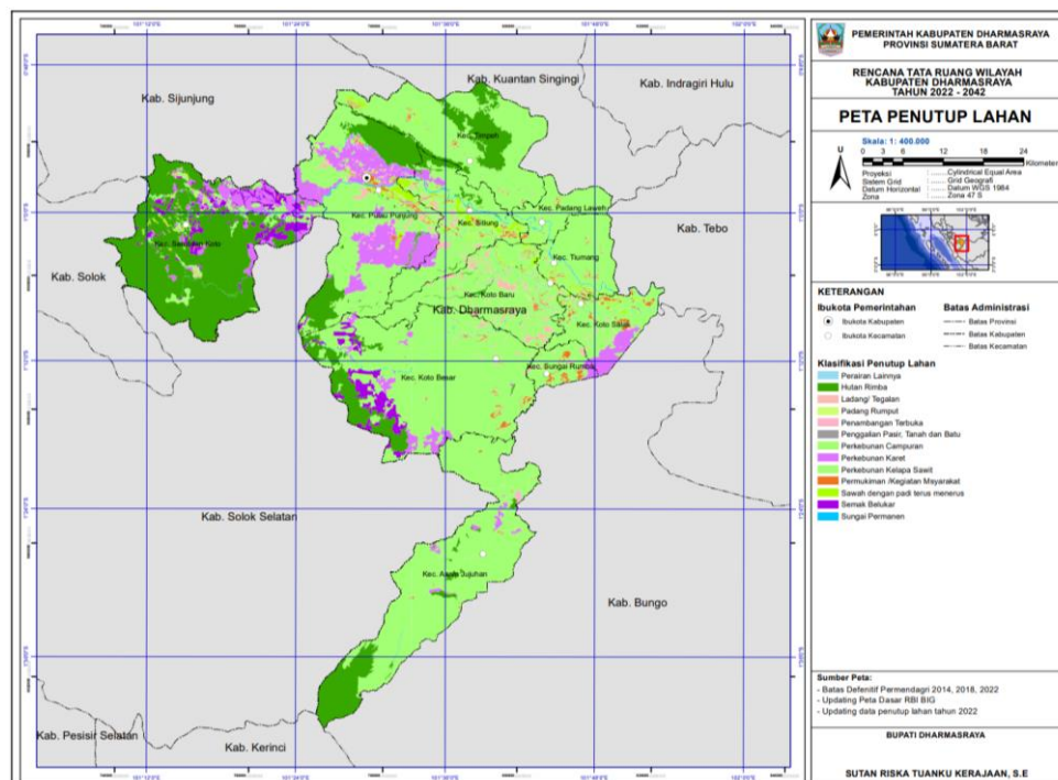
Gambar 2-8 Peta Tutupan Lahan Kabupaten Dharmasraya
