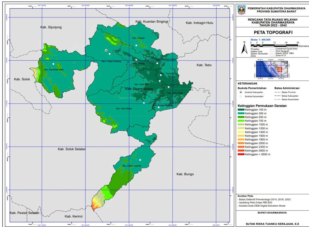
Gambar 2-2 Peta Topografi Kabupaten Dharmasraya
